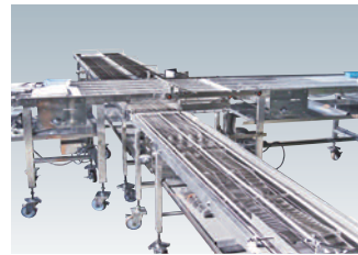
网格传送带
